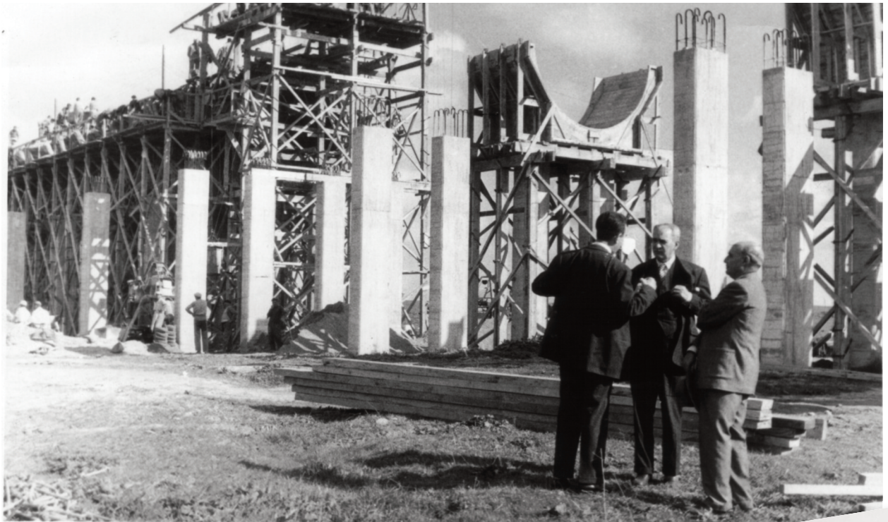
Obras de construcción del sifón-viaducto del Guadaira. Fuente: Archivo G.T. RMHSA, CGT.A
